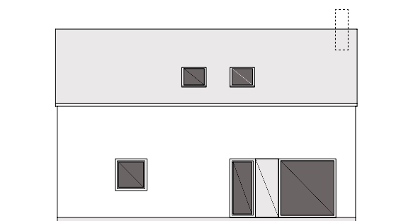
POHLED P4
