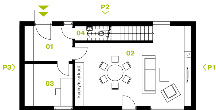
PŮDORYS PŘÍZEMÍ P4
