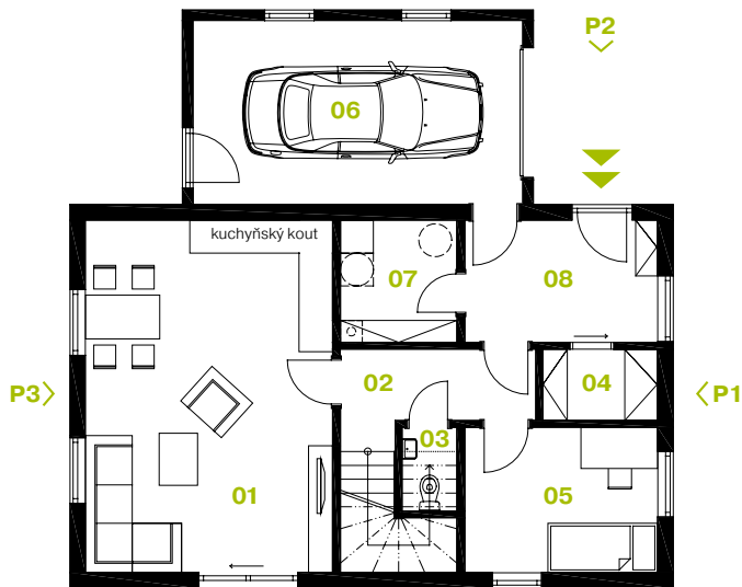
PŮDORYS PŘÍZEMÍ
